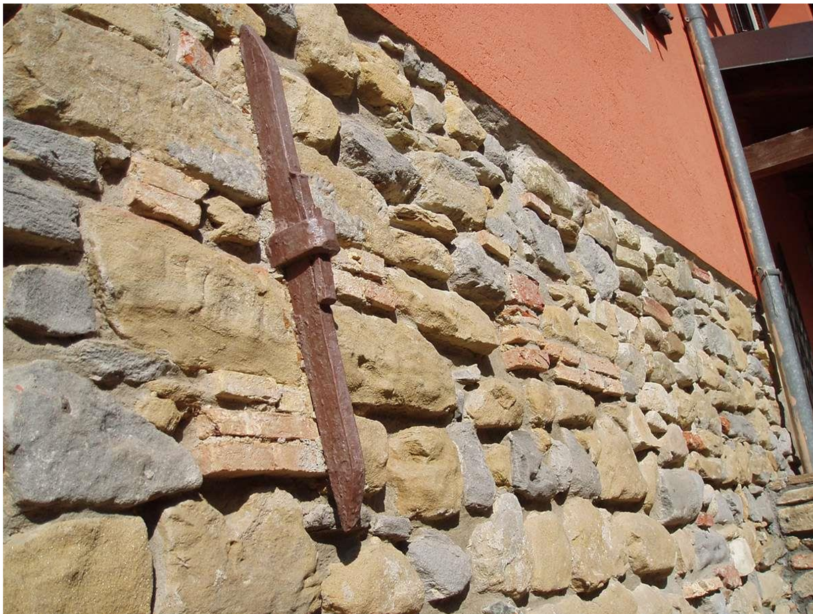
muro-di-contenimento-in-Pietra-di-Molera 1
